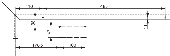
2 - Deurbladmontage niet-scharnierzijde
